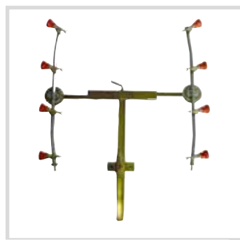
RAMPE ARRIÈRE DE PULVÉRISATION POUR VIGNOBLES (6-8-10 buses)
